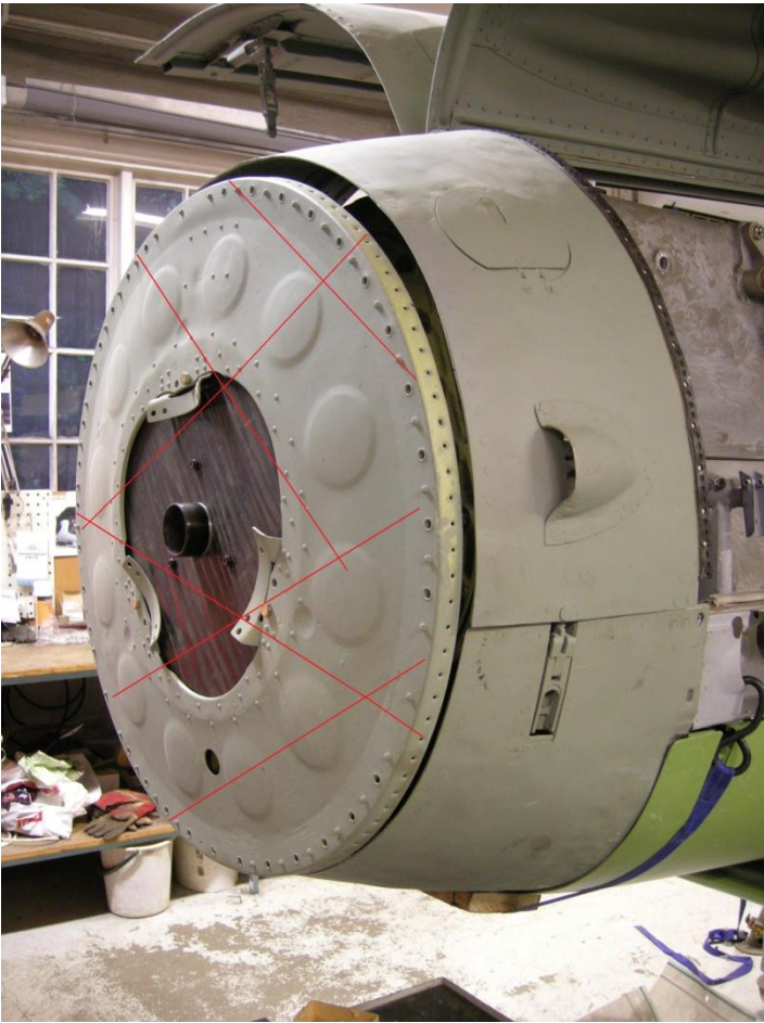
Reparerte originale fremre deksler G10 for stor olje tank
